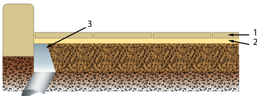
1 - Produits de dallage 2 - Lit de pose en sable 3 - Évacuation
